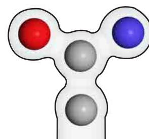
Asparagine
