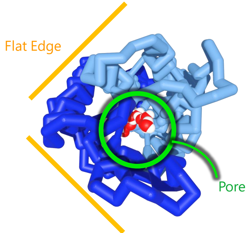
Monomer
